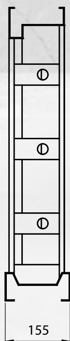
Vista lateral
